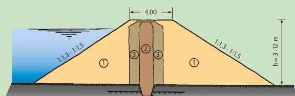
Teichdämme – Neue Bauart
