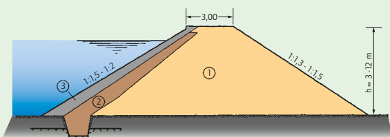
Teichdämme – Alte Bauart
